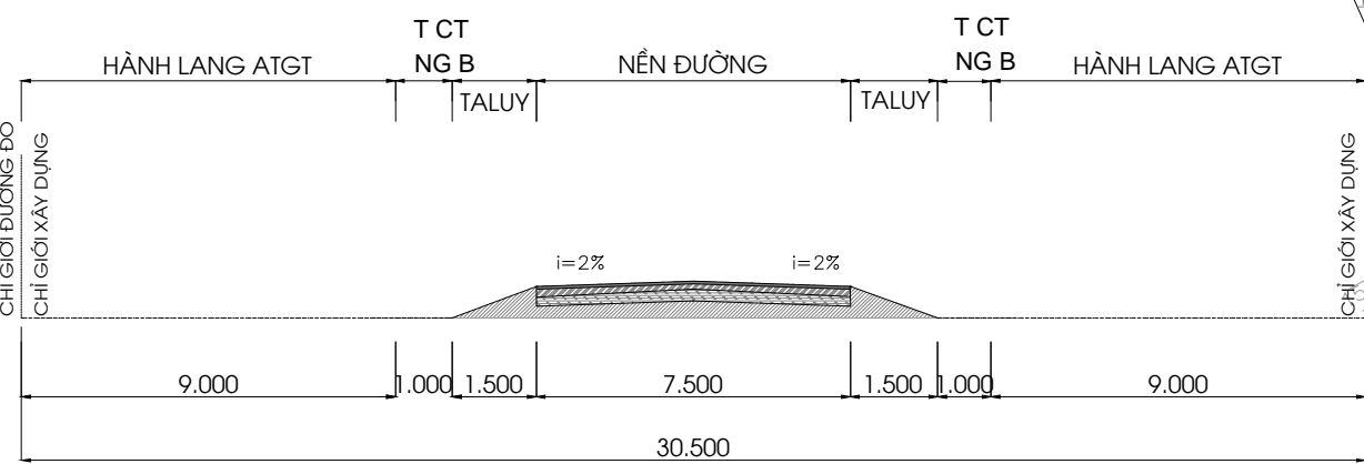
MẶT CẮT 3-3 (ĐT.573.A)
