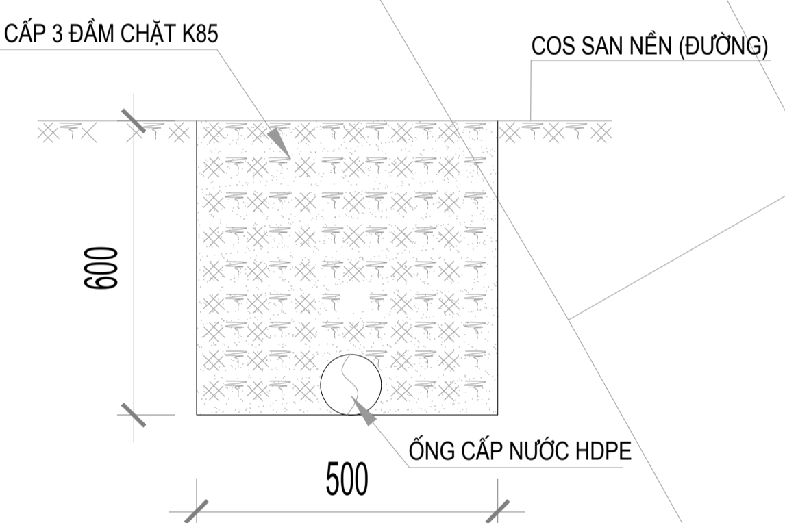
MẶT CẮT NGANG ĐẶT ỐNG CẤP NƯỚC
