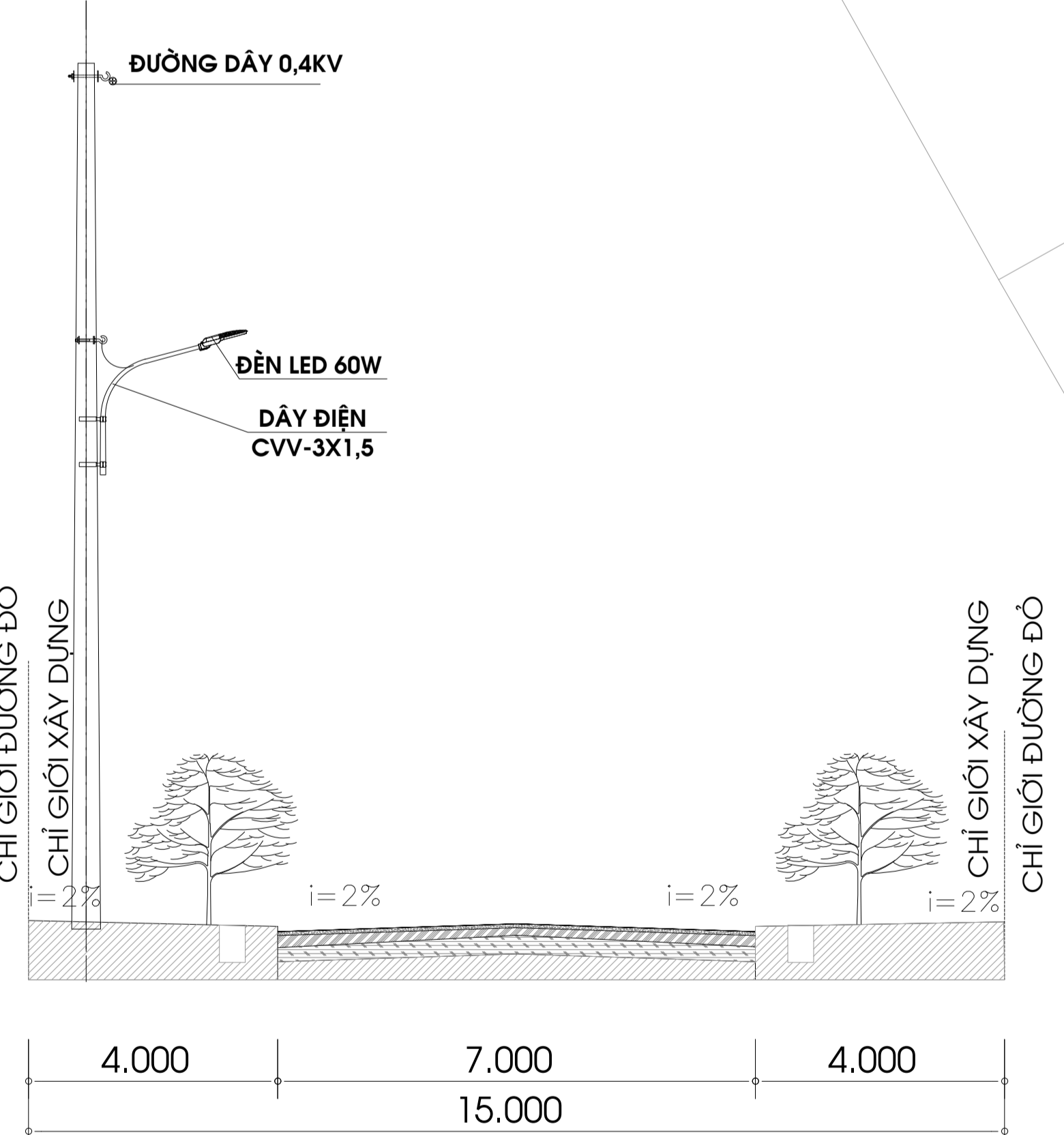
MẶT CẮT 2-2
